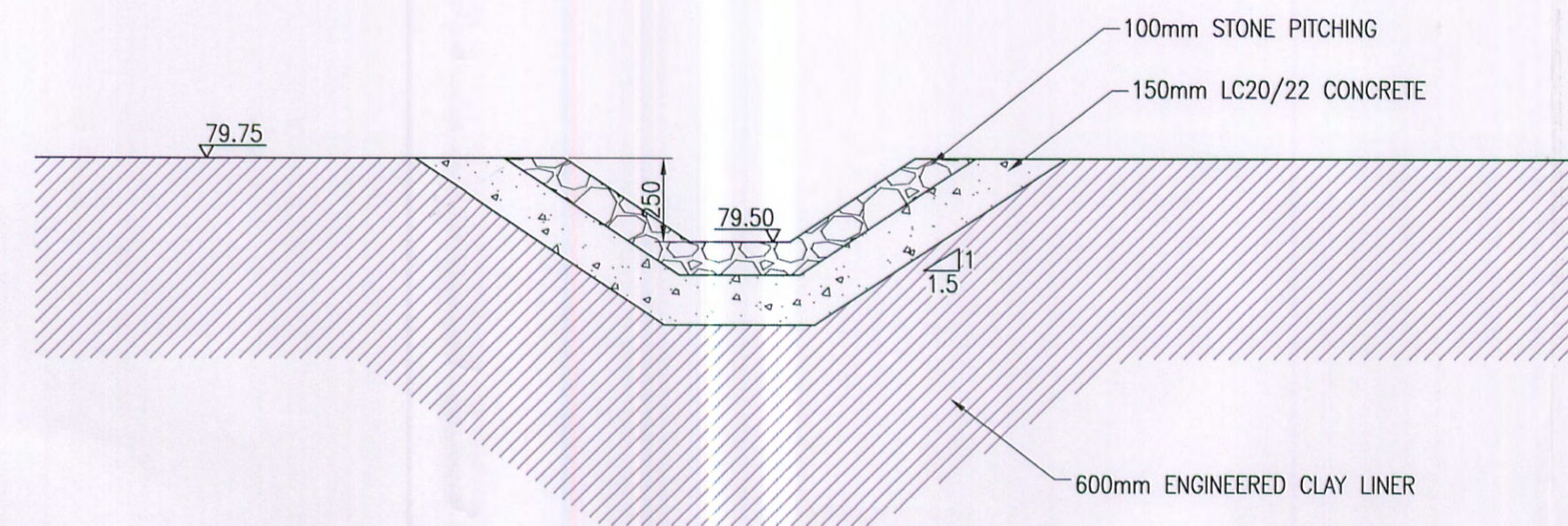
SECTION D-D
